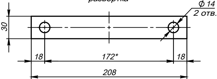
Поз.10 (Полухомут) развертка
