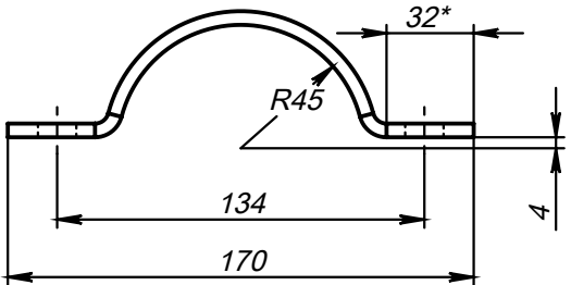
Поз.10 (Полухомут) развертка
