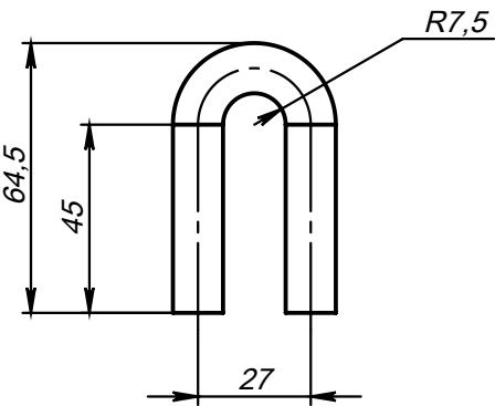
Поз.2 (Ушко) 1 : 2
