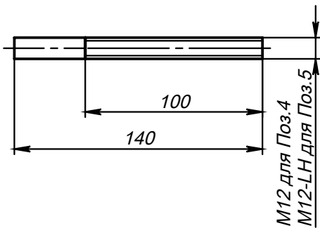
Поз.4 и Поз.5 (Шпилька)
