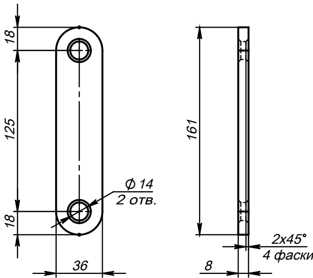
Поз.9 (Серьга)
