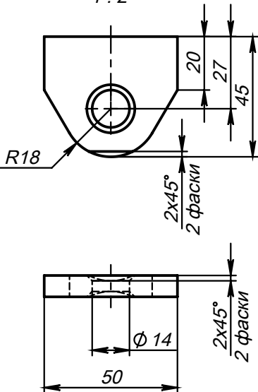
Поз.1 (Проушина) 1 : 2
