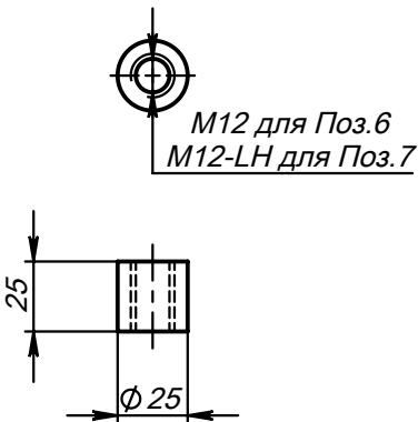
Поз.6 и Поз.7 (Гайка)
